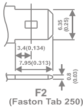
F2 (Faston Tab 250)
